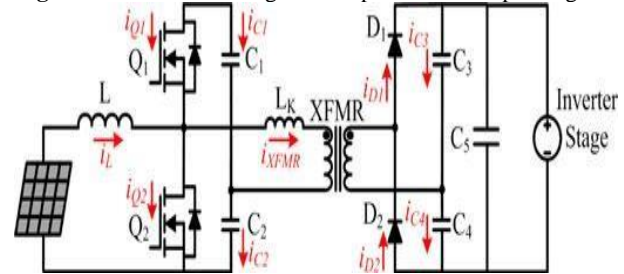
Fig. 3. IBR Converter
